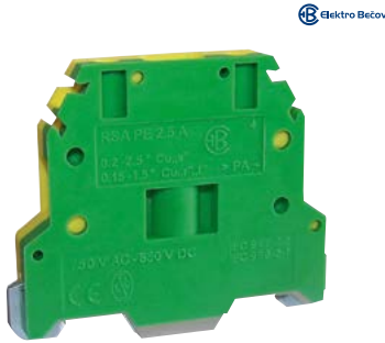
Svorka řadová RSA PE šroubovací, montáž na lištu DIN, krytí IP 20, barva zelenožlutá
