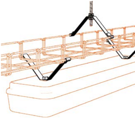
Držák žlabu ARKYS DZM 3/150 pro zavěšení kabelových žlabů šířky 150 mm na závitové tyče M8, lze jej využít i jako nosný prvek pro instalaci různých typů svítidel, galvanicky zinkováno
