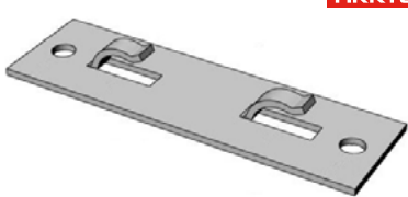
Držák žlabu nástěnný ARKYS DZM 10 pro použití pro více typů instalace svislé i vodorovné montáže, především u kovových konstrukcí, na které se dá upevnit šrouby, případně navařením, galvanicky zinkováno
