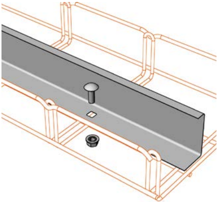
Spoj přepážky ARKYS SPM 1 k upevnění přepážky do libovolného místa v celé šíři žlabu, galvanicky zinkováno, sada: šroub vratový M6×16, matice límcová M6, 10 ks/bal., cena za ks
