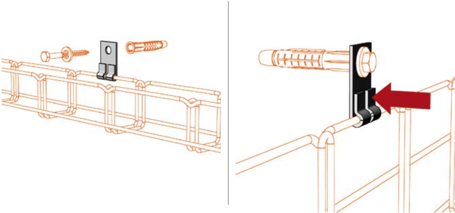
Držák žlabu nástěnný ARKYS DZM 8 pro ukotvení kabelových žlabů v nástěnné montáži přímo do svislých částí stavby, max. doporučená šíře žlabu je 50 a 100 mm, galvanicky zinkováno, 10 ks/bal., cena za ks
