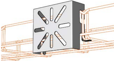
Držák rozvodných krabic ARKYS DZM 1 pro upevnění rozvodných krabic a ostatních prvků (zásuvek, vypínačů atd.) přímo na kabelovou trasu, maximální nosnost držáku 5 kg, galvanicky zinkováno
