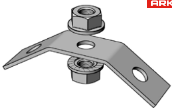
Držák závěsných lanek ARKYS DZM 15 pro ukotvení závěsného lanka na závitovou tyč, pro pomocné lanové zavěšení žlabů, galvanicky zinkováno
