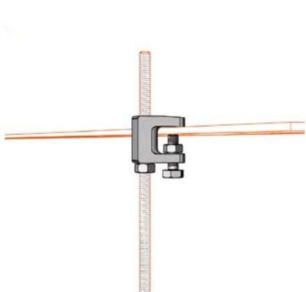
Držák závitové tyče ARKYS DZM 9 pro ukotvení závitových tyčí M8 prostorové montáže zavěšením na I profil, max. doporučené zatížení držáku je 120 kg, galvanicky zinkováno
