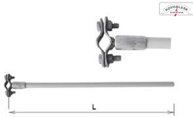
Tyč izolační IZT-J930 pro uchycení jímací tyče, materiál GFK, délka 930 mm
