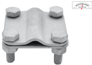
Svorka zemnicí SR 03 K pro křížové spojení a souběžné zemnicí pásy a kruhového vodiče hromosvodu, materiál FeZn, rozměry 55×55 mm
