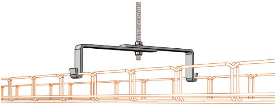
Držák žlabu nastavitelný ARKYS DZM 4 pro zavěšení kabelových žlabů šířky 200–300 mm na závitové tyče M8, nelze použít v kombinaci s vikem žlabu, galvanicky zinkováno
