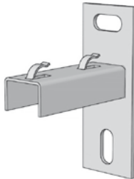
Nosník žlabů ARKYS NPZM nástěnné nosné prvky pro montáž kabelové trasy, galvanicky zinkováno, plech tloušťky 2 mm (základna 5 a 6 mm), bezšroubové úchyty
