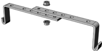
Držák žlabu nastavitelný ARKYS DZM 4 pro zavěšení kabelových žlabů šířky 200–300 mm na závitové tyče M8, nelze použít v kombinaci s vikem žlabu, galvanicky zinkováno
