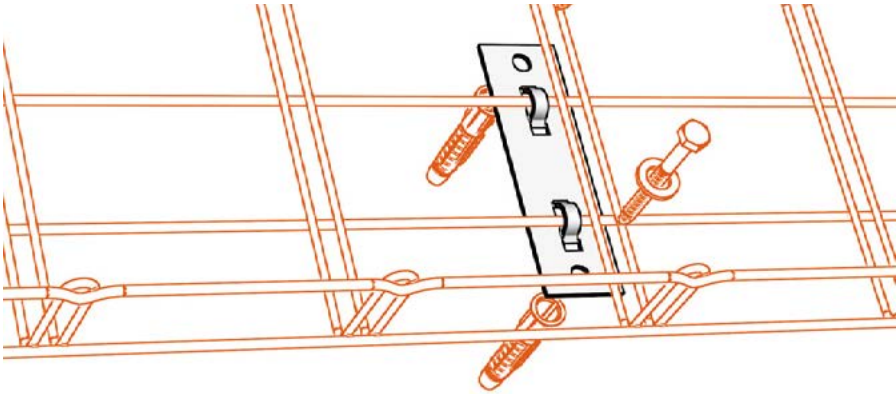
Držák žlabu nástěnný ARKYS DZM 10 pro použití pro více typů instalace svislé i vodorovné montáže, především u kovových konstrukcí, na které se dá upevnit šrouby, případně navařením, galvanicky zinkováno
