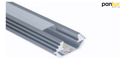
Profil ALU přisazený speciální mléčný difuzor, materiál kov + plast, včetně spojovacího materiálu, délka 2 m, pro šířku pásku 10 mm, speciální
