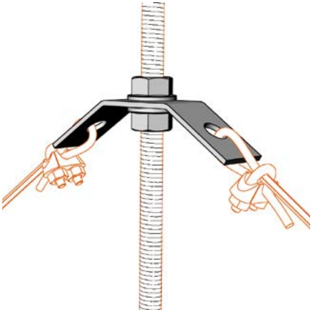
Držák závěsných lanek ARKYS DZM 15 pro ukotvení závěsného lanka na závitovou tyč, pro pomocné lanové zavěšení žlabů, galvanicky zinkováno
