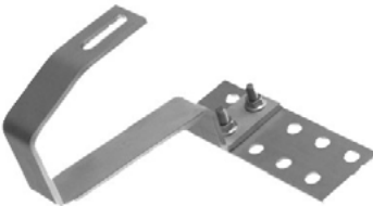
Hák kombinovaný (univerzální) NH2 kombinovaný, materiál nerezová ocel A2, univerzální
