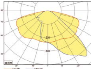
křivka svítivosti
