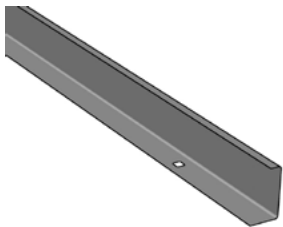
Přepážka žlabu ARKYS KPZM 50 pro oddělení silno/slaboproudého vedení nebo pro větší přehlednost, nerezová ocel A2, výška 43 mm, tloušťka plechu 0,8 mm, hmotnost 1,2 kg, délka 2 m
