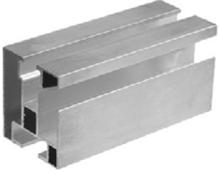
Profil hliníkový HNP1 rozměry 40×45 mm, délka 6 300 mm
