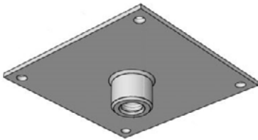
Držák závitové tyče ARKYS DZM 2 pro ukotvení závitových tyčí M8 při prostorových montážích do stropu, galvanicky zinkováno
