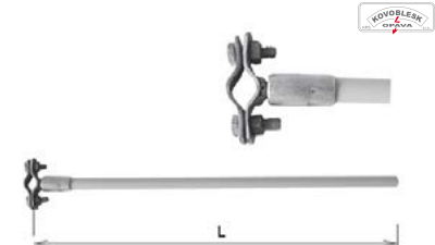
Tyč izolační IZT-J430 pro uchycení jímací tyče, materiál GFK, délka 430 mm
