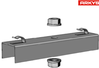
Podpěra žlabů ARKYS PZM pro uchycení na závitové tyče, galvanicky zinkováno, plech tloušťky 1 mm, bezšroubové úchyty
