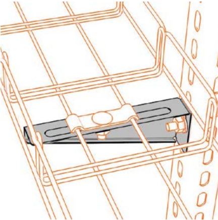
Nosník žlabů univerzální ARKYS NZMU nosné prvky pro montáž jedné nebo více kabelových tras nebo vodo-topo instalací, galvanicky zinkováno
