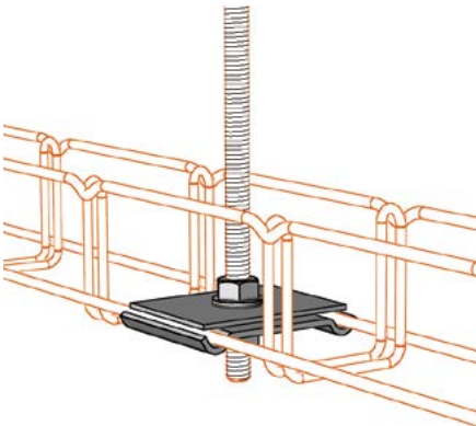
Držák žlabu ARKYS DZM 13 pro prostorovou instalaci kabelových žlabů na závitové tyče M8, galvanicky zinkováno, 10 ks/bal., cena za ks
