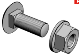
Spoj přepážky ARKYS SPM 1 k upevnění přepážky do libovolného místa v celé šíři žlabu, galvanicky zinkováno, sada: šroub vratový M6×16, matice límcová M6, 10 ks/bal., cena za ks
